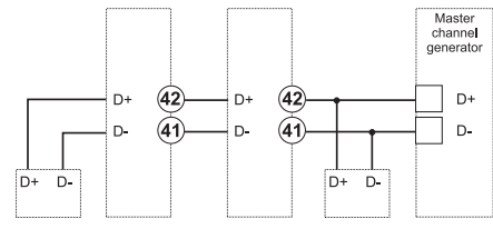
Fig. 30 Dupline port
