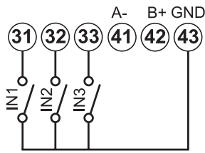
Fig. 28 Digital inputs
